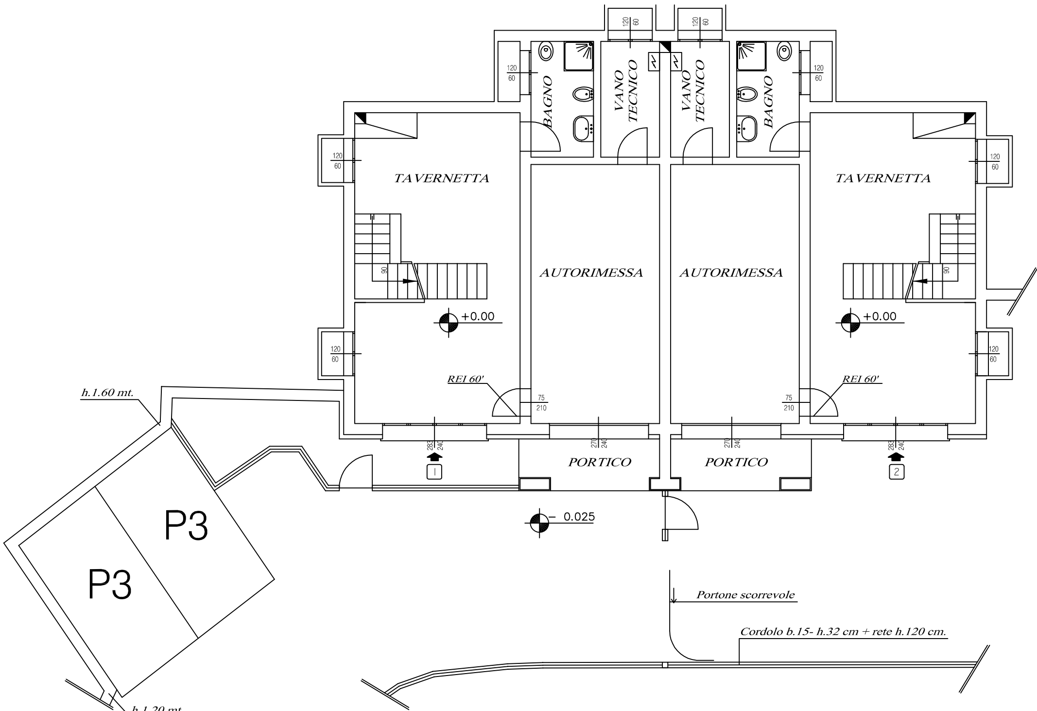
PIANTA PIANO TERRA h.2,70 m.
